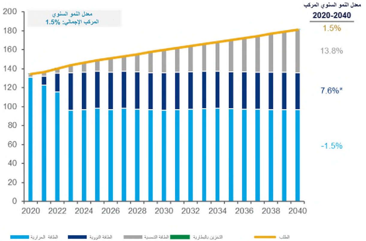
الشكل (٣): توقعات الطلب والعرض للطاقة في دولة الإمارات (تيراواط في الساعة)
