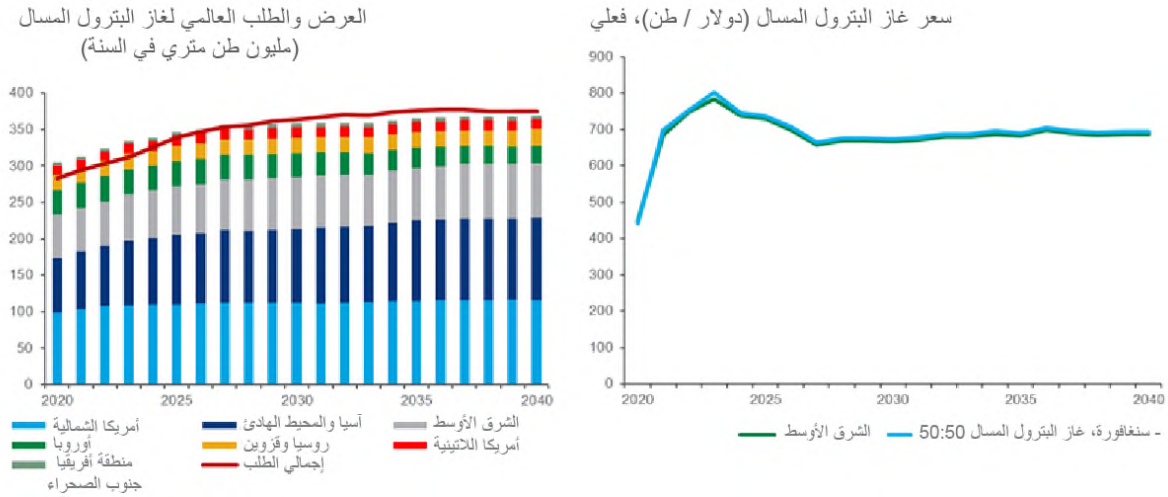
الشكل (١٢): التوقعات العالمية لغاز البترول المسال (الطلب والعرض والتسعير)، مليون طن متري في السنة، طن / دولار
