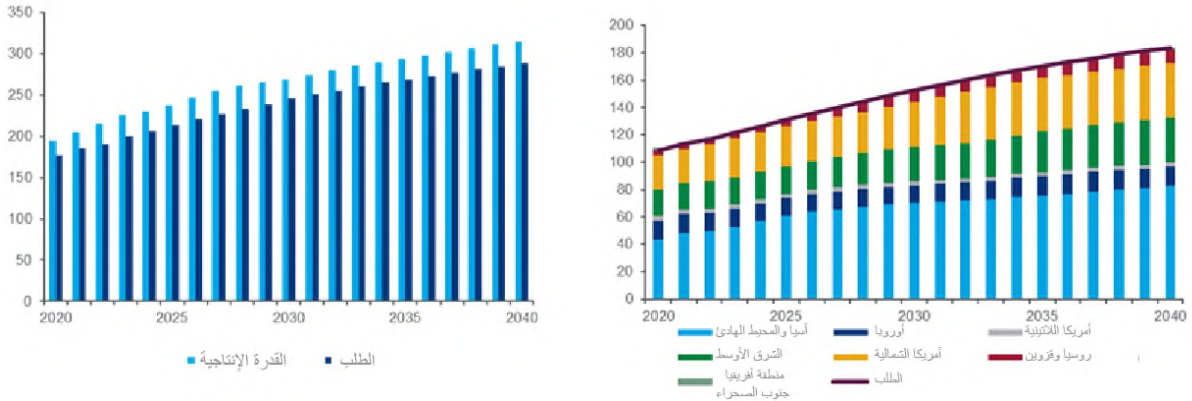
الشكل (١٠): التوقعات العالمية للإيثيلين والبولي إيثيلين (العرض والطلب)، مليون طن متري في السنة
