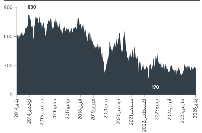
الشكل 17: النافثا - البولي إيثيلين عالي الكثافة
