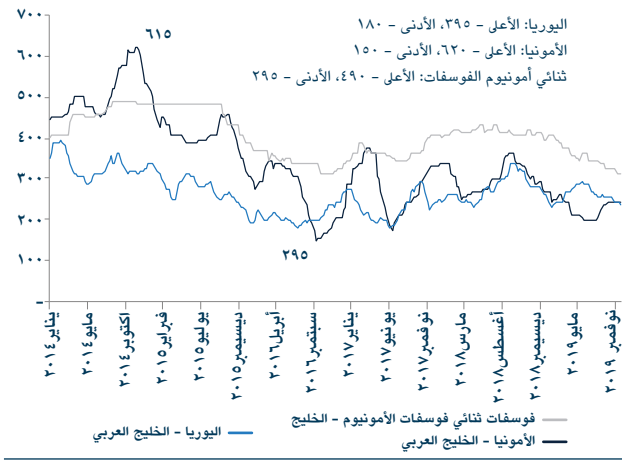
الشكل ١٤: الأمونيا واليورينا وثنائي أمونيوم الفوسفات
